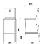
空スタンド椅子 寸法図
