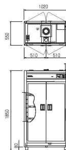
ESN-2DB (両面扉式)
