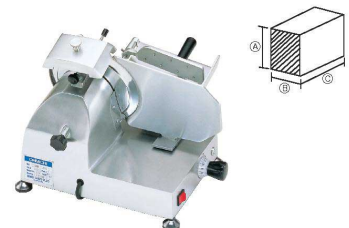
6 牛タンスライサー OMS-230 [EHSL-45]
