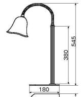
ミニヒートランプ寸法図 (mm)
