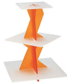
⑥ スタンド Cod.308 [NSVS-05] 組 17-0876-0601 ¥84,000 サイズ:400×400×H530 プレート:1段目/400×400 2段目/300×300 3段目/220×220
