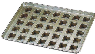
⑦ シリコン加工 フォーマル型天板 (35ヶ取) (WTV-14) 1-1126-0701 ¥39,500 545×395×H54 単品寸法 (A) (B) (H) 内 45×45×30
