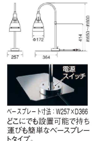
9 ランプウォーマー ベースプレート式 SL-25BA 〈NLV-39〉 1-1675-0901 ¥150,000 257×約366~600×H約650~800 電源：単相100V 50/60Hz 消費電力：250W ランプ仕様：赤外線ランプ250W(口金サイズE26) ベース：257×366 ランプ可動範囲：200~400 質量：4.9kg
