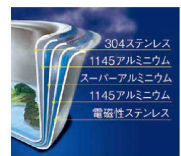
全面5層構造
