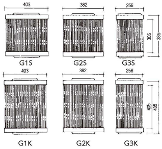
KG-5C ローストックK-5CとグリッドバーG1K・G3Kの組合わせ。
