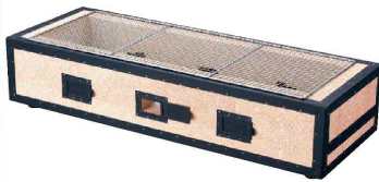
1 炭火バーベキューコンロ BQ-22号 (8~12人用) 〈DBC-39〉 1-0773-0101 ¥108,000 920×350×H200 質量25kg 付属品:焼アミ1枚 材質:けいそう土
