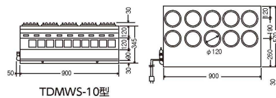
TDMWS-10型
