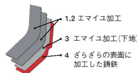
黒マットエマイユ加工の構造
