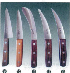
日本鋼解体包丁 ⑨ 骨スキ 角(片刃) [CHRA-13] 18-0148-0901 ¥12,500 全長:265 刃渡:150 背厚:2.5
