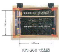
NN-260 寸法図
