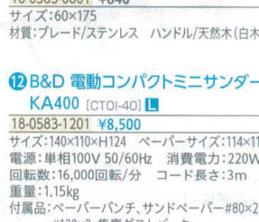
12 B&D 電動コンパクトミニサンダー KA400 [CTOI-40] 国産 18-0583-1201 ¥8,500 サイズ: 140×110×H124 ペーパーサイズ: 114×114 電源: 単相100V 50/60Hz 消費電力: 220W 回転数: 16,000回転/分 コード長さ: 3m 重量: 1.15kg 付属品: ペーパーパンチ、サンドペーパー#80×2、#120×2、集塵ダストバック ●低重心設計で、自由な操作性を実現し、高速振動とハイパワーで効率的な研磨が可能です。 ●握りやすいソフトラバーグリップで長時間の作業も快適です。 ●市販のサンドペーパーも使用出来ます。
