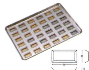
④ シリコン加工 センチュリー型 天板 小 36連 [DKTV-65] 18-0648-0401 ¥36,500 サイズ: 545×395×H33 出来上がり寸法: A49×B26×H11 材質: プリキ/シリコン樹脂加工
