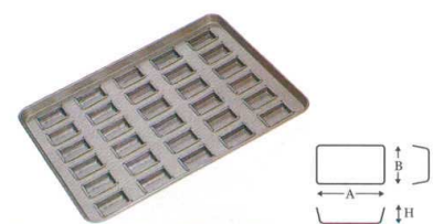
⑧ シリコン加工 トロフィー型 天板 30連 [DKTV-67] 18-0648-0801 ¥35,000 サイズ: 545×395×H38 出来上がり寸法: A61×B36×H15 材質: プリキ/シリコン樹脂加工
