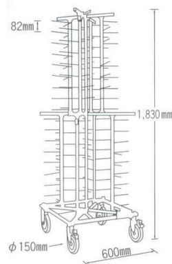
② プレートディスペンサー (移動式) ジャックスタック JS072
