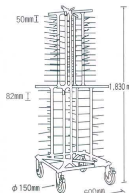
③ プレートディスペンサー (移動式) ジャックスタック JS088
