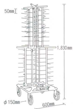
① プレートディスペンサー (移動式) ジャックスタック JS104
