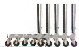
18-0082-1201 ¥72,100 外寸: 739×550×H1,700 重量: 27.2kg 材質: 床板/ポリプロピレン、棚板/フレーム/スチール(塗装仕上げ) キャスター: ゴム製 φ125 (固定×2輪 1輪ストッパー付) (自在×2輪 2輪ストッパー付) 耐荷重: 300kg ●一般的なカートンサイズに合わせたデッキ面サイズです。滑り止めもそれに合わせて効果的に配置しています。 ●背面4箇所の緩衝材により、壁際への設置でも金属フレームが直接接触しません。 ※ネスティングは5台までを推奨
