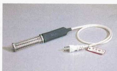
⑭ チューフィンングヒーター 電気式 (4422800) 外寸: 本体長さ/220mm コード長さ: 60cm 電源: 単相 100V 280W
