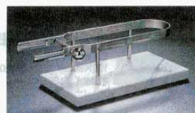
㉓ ハムホルダー 大理石 外寸: 600×245×H190mm (1458300) 大理石台 480×245mm ホルダー 全長: 600×H140mm 最大幅: 150mm (中心) 最小幅: 130mm (中心)
