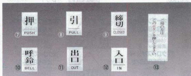
点字サイン 60×40×厚さ2mm ⑦ TS641-1 押(PUSH) (7674600) ⑤ ⑧ TS641-2 引(PULL) (7674700) ⑤ ⑨ TS641-3 締切(CLOSED) (7674800) ⑤ ⑩ TS641-5 呼鈴(BELL) (7674900) ⑤ ⑪ TS641-6 出口(OUT) (7675000) ⑤ ⑫ TS641-7 入口(IN) (7675100) ⑤ 点字サイン 120×50×厚さ2mm ⑬ TS126-1 ご用の方はこのボタンを押して下さい。 (7675200) ⑤
