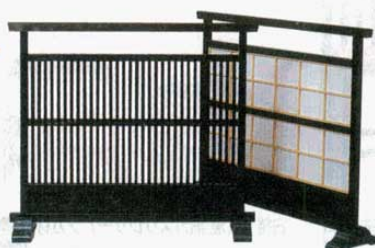
② 衝立 千本格子 1,050×250×H1,000mm (3841200) 材質：ツガ材 ※裏面は障子張りです。 ※障子は取りはずしできます。
