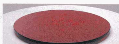
③ ターンテーブル (メラミン化粧板・ソフトエッジ巻) TT4-750 φ 750 (435) × H52mm (6479300) TT4-900 φ 900 (435) × H52mm (6479400) TT4-1200 φ 1,200 (580) × H52mm (6479500) 天板厚: 30mm
