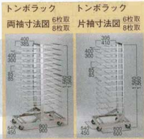
⑤ トンボラック 26枚差 天板・食パン用 鉄製 EBM (8804000) 940×550×H1,600mm 車輪：φ100×4自在 (2輪ストッパー付) ※シルバーコーティング仕上げ フレーム間隔：85mm ●フレームは1段おきに取りはずしが出来、天板はもちろん、背の高い食パンケースも収納出来ます。
