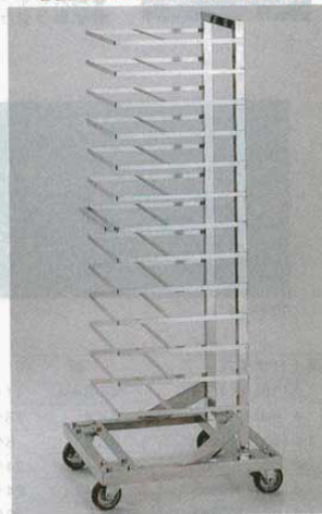
② トンボラック 片袖 (13枚差) 18-8 EBM 6枚取用 (4547400) 8枚取用 (4547500) 車輪：φ100×4自在 (2輪ストッパー付)
