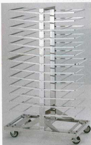
① トンボラック 両袖 (26枚差) 18-8 EBM 6枚取用 (4547200) 8枚取用 (4547300) 車輪：φ100×4自在 (2輪ストッパー付)
