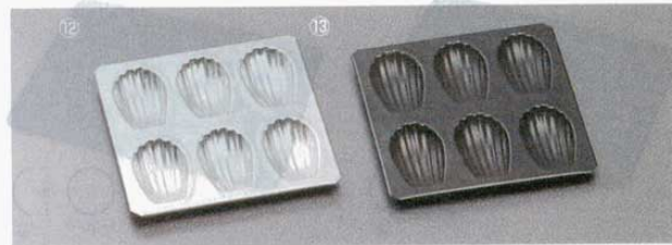
⑫マドレーヌ 77151 マトファー (スズメッキ) 6ヶ取 (2589800) 196×190mm (1ヶ当り80×40mm) ⑬マドレーヌ 677152 マトファー (テフロン加工) 6ヶ取 (2590200) 196×190mm (1ヶ当り80×40mm)
