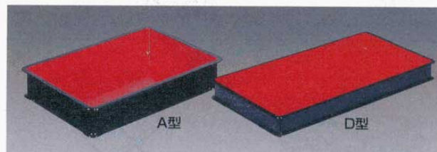
⑫番重 朱塗 ABS サンコー A型 外寸 574×388×H97mm (4860500) ㊞ 内寸 534×348×H90mm B型 外寸 574×388×H67mm (4860600) ㊞ 内寸 534×348×H60mm D型 外寸 697×343×H64mm (4860700) ㊞ 内寸 662×318×H53mm 中型 外寸 487×336×H75mm (4860800) 内寸 453×302×H63mm
