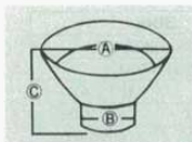
① ストレーナープレス 24100 鋼タイプ INOX Gefu (7271800) ボール：内径 190mm 高さ 80mm 全長 390mm 全高 190mm
