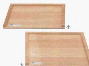
⑤ のし板 三方枠付 木製 大 600×600×H25mm (0059200) 小 540×420×H25mm (0067900) 材質: アラスカ松 ※粉の飛びちりを防ぎます。
