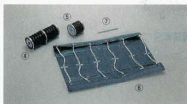
④ 空気バネ(完成) 大 (7004800) φ105×280mm ①～③各共通 ⑤ 空気バネ(完成) 小 (7004900) φ105×135mm ①～③各共通
