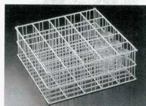
① グラスラック EBM 5×5 (475×475mm) ゴブレット用 高さ 185 幅 86 奥行 165 (0985500) カクテル、 ブランド用 130 86 110 (0985700) シャンパン用 140 86 120 (0985900)
