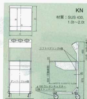
③ ラック・トレイディスペンサー KN5245-T4 リフト型
