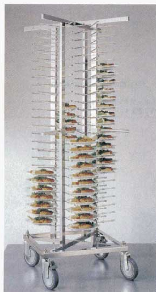
③ ディッシュスタック 100 ユニバーサル EBM (4589100)
