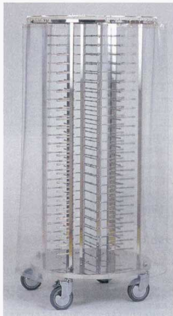
① ディッシュスタック 100 カーテン式(丸型) EBM (6201100) φ785×1,790mm カバーの取り付け、取りはずしの煩わしさを解消しました。従来の角型から丸型にする事により、全体を均一にカバーします。カーテン式ですので皿の出し入れもスムーズにできます。 ※φ18cm～33cmの皿が使用できます。 ※キャスターφ150mm 4輪自在(内2ヶストッパー付)
