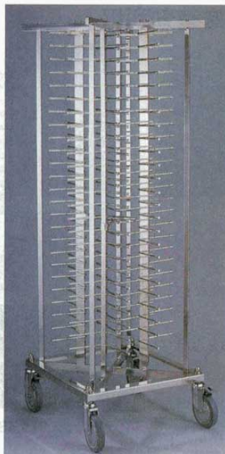
② ディッシュスタック 100-4P EBM (4869900) 4本の柱を入れたことにより、従来のEBMディッシュスタック100に比べ、安全性(ガード)と安定性に優れ、移動も容易になりました。 ※φ18cm～33cmの皿が使用できます。 ※キャスターφ150mm 4輪自在(内2ヶストッパー付)
