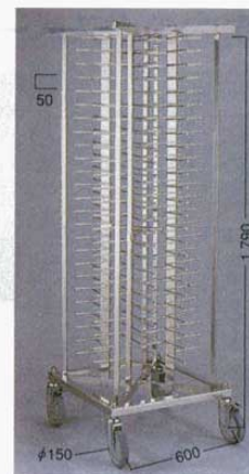
② ディッシュスタック 100-4P EBM (4869900) 4本の柱を入れたことにより、従来のEBMディッシュスタック100に比べ、安全性(ガード)と安定性に優れ、移動も容易になりました。 ※φ18cm～33cmの皿が使用できます。 ※キャスターφ150mm 4輪自在(内2ヶストッパー付)
