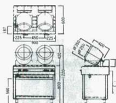
② ロータリーシェフ RC-2 スタンド型 ガス式 外寸：900×600×H1,220mm
