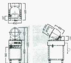
① ロータリーシェフ RC-1 スタンド型 ガス式 外寸：450×600×H1,220mm
