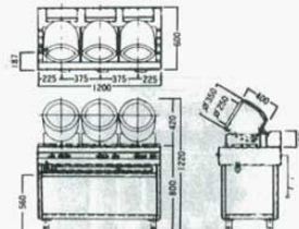
③ ロータリーシェフ RC-3 スタンド型 ガス式 外寸：1,200×600×H1,220mm
