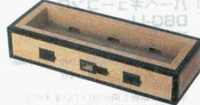
④ バーベキューコンロ BQ22号 炭用 (6559700) 外寸: 930×350×H210mm 内寸: 800×215×H115mm 重量: 25kg 付属品: 焼きアミ
