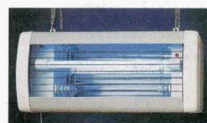
⑫ 電撃殺虫器 TSH-20210 (片面配光型) (5184000) 外寸: φ800×320×H360mm チェーン70cm 定格電圧: 100V 捕虫ランプ20W×2灯 有効面積: 200~300㎡ OUT DOOR 重量: 19kg 用途: 店舗出入口 ※店内側や呼び寄せたくない側への光をカット
