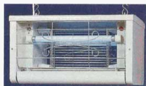
① 電撃殺虫器 NS-100 (6249600) 外寸: 486×304×H270mm チェーン70cm 定格電圧: 100V 10W×2灯 有効面積: 30~50㎡ IN DOOR 重量: 9.5kg
