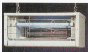
② 電撃殺虫器 NS-150 (1188700) 外寸: 592×304×H270mm チェーン70cm 定格電圧: 100V 15W×2灯 有効面積: 60~100㎡ IN DOOR 重量: 11kg
