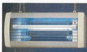
⑪ 電撃殺虫器 TSS-20210 (5183900) 外寸: φ800×320×H360mm チェーン70cm 定格電圧: 100V 捕虫ランプ20W×2灯 有効面積: 200~300㎡ OUT DOOR 重量: 18kg 用途: 店舗出入口 軒下
