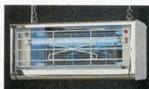
③ 電撃殺虫器 NS-150DX (1188600) (ステンレスタイプ) 外寸: 592×304×H270mm チェーン70cm 定格電圧: 100V 15W×2灯 有効面積: 60~100㎡ IN DOOR 重量: 11kg
