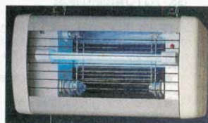
⑩ 電撃殺虫器 TSS-15210 (6250100) 外寸: φ656×320×H360mm チェーン70cm 定格電圧: 100V 捕虫ランプ15W×2灯 有効面積: 150~300㎡ OUT DOOR 重量: 17kg 用途: 店舗出入口 軒下
