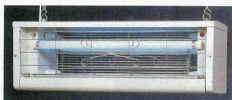
⑤ 電撃殺虫器 NS-300 (1188500) 外寸: 786×304×H270mm チェーン70cm 定格電圧: 100V 30W×2灯 有効面積: 100~200㎡ IN DOOR 重量: 12.5kg
