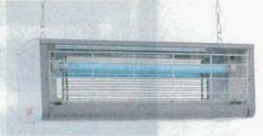
⑦ シュアー屋内用電撃殺虫器 GK-5010DX (1127200) 外寸: 786×304×H270mm 材質: ステンレス ●取付高さ床1.8m以上 ●二重安全装置付き(虫受け皿、保護カバー) ●チェーン吊り下げ式
