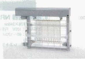
⑩ シュアー屋外用電撃殺虫器 GK-7010Z (1128600) 外寸: 876×330×H680mm ●耐久性に優れた高級塗装仕上げ ●取付高さ地上3.5m以上 ●有効面積200~400㎡ ※設置条件により別売の専用取り付け金具⑪~⑬が必要です。
