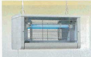
③ シュアー屋内用電撃殺虫器 GK-2020Y (1127300) 外寸: 486×304×H270mm ●メラミン焼き付け塗装の側板 ●取付高さ床1.8m以上 ●二重安全装置付き(虫受け皿、保護カバー) ●チェーン吊り下げ式
