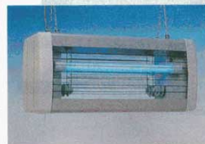
⑧ シュアー屋外用電撃殺虫器 GK-6100Z (1128400) 外寸: 800×320×H364mm ●耐久性に優れた高級塗装仕上げ ●取付高さ地上1.8m以上 ●二重安全装置付き(虫受け皿、保護カバー) ●チェーン吊り下げ式
