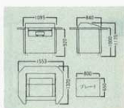
① ステーキテーブル S-111 (1244300) キャスター：自在φ100mm×4（2輪ストッパー付）
