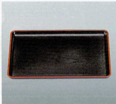
[A] ケヤキ会席盆 黒天朱(ノンスリップ加工) 68216-804 尺1寸 1,500円 50入 (33×24×2cm) 68217-804 尺2寸 1,850円 40入 (35.5×25.6×1.8cm) 68218-804 新尺2寸 2,100円 40入 (37×29×1.8cm) 68219-804 尺3寸 2,150円 40入 (39.1×28×1.8cm) 68220-804 尺4寸 2,600円 40入 (42.5×30.1×1.8cm) 68221-804 尺5寸 3,300円 30入 (45.4×31.6×2cm) 68222-804 尺6寸 4,200円 20入 (48.2×33×2cm)
