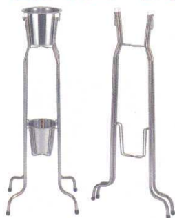
① フラスタンド 折りたたみ式 18-8 8040400 S-1 480×340×H1,240 花入れ：上 φ220×φ170×H205 下 φ174×φ135×H165
