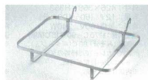
⑦ブレードバスケットホルダー 2127 1626400 18-8ステンレス 外寸：508×432×H115
