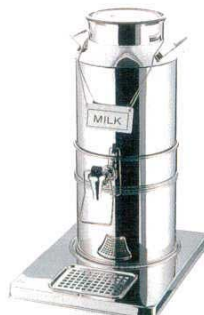
③ ミルクディスペンサー L UK 7475400 370×480×H635 容量：15ℓ 材質：18-8ステンレス
