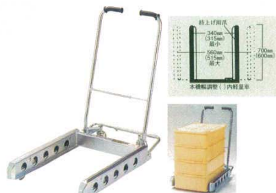
⑰ ビックカート 軽量車 (積載能力: 80kg用) 3049000 キャスター: φ75 ゴム製 重量車 (積載能力: 150kg用) 3049100 キャスター: φ100 ゴム製 ※床置きコンテナ・BOXをそのまま手付けず くい上げ、手軽に目的地に移動出来ます。
