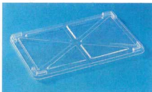
② 番重用蓋 クリスタル サンコー A・B型用 外寸: 590×401×H30 4860400 10 ※特殊樹脂
