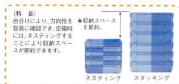
①NF-M33 外寸：648×417×H155 内寸：602×377×H145 容量：32ℓ 5637000 ②NF-M39 外寸：532×370×H260 内寸：486×330×H254 容量：39ℓ 5637100
