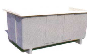
③ジャンボタンク 910S 8433300 外寸：1,650×1,130×H710 内寸：1,530×1,010×H600 容量：約910ℓ 本体重量：29kg 材質：FRP 規格色：ホワイト・グレー 脚間隔：920mm
