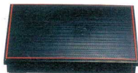
⑫ 松花堂弁当 干筋 (仕切別) 黒天朱 R3 377×260×H65 2507000 材質: ABS樹脂
