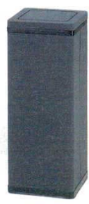
㉔ ロータリー屑入 RSL-208N スエード 外寸：240×240×H600 6573800 材質：亜鉛メッキ銅板アクリル塗装 重量：4.5kg 容量：16ℓ 付属品：中箱付
