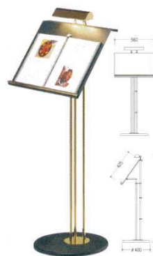
④メニュースタンド ルミエ 7700100 パネルサイズ: 560×H425 材質: スチール製 電源: 単相110V・60W ランプ: 30Wクリアスペース球 (E-17) 2灯、2.5mコード付
