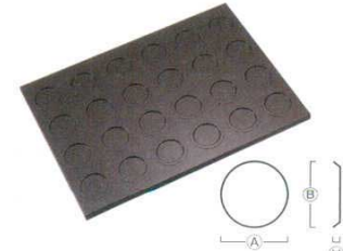
⑫天板 ラング・ド・シャ丸型 テフロン加工 (24ヶ取) 6739400 545×395×H20 単品寸法: A70 B65 H4.5
