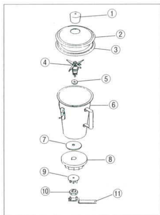
本体側部品
