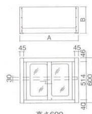
高さ600 (棚板1枚)
