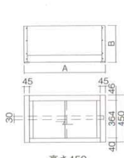
高さ450 (棚板1枚)
