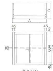
高さ750 (棚板1枚)
